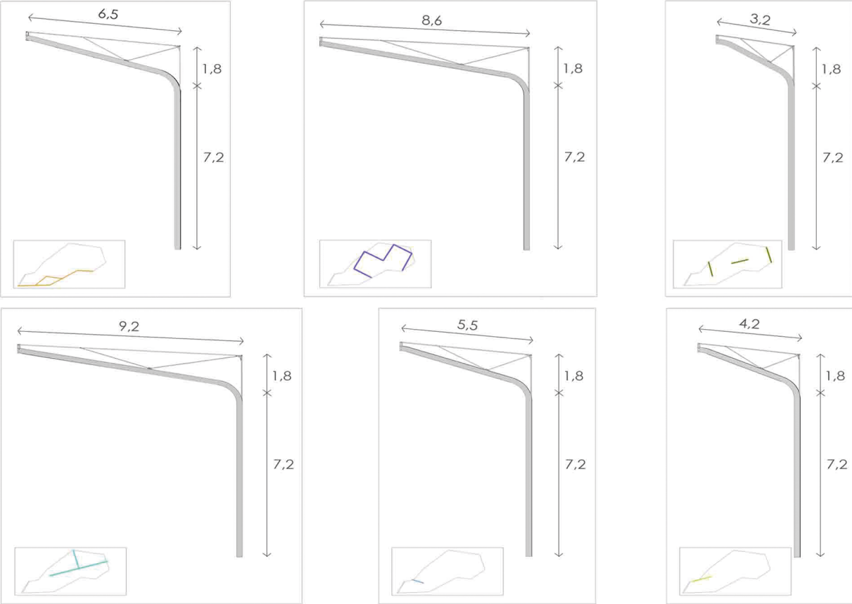
Katalogoa (Estalkiak) Catálogo (Cubiertas)
