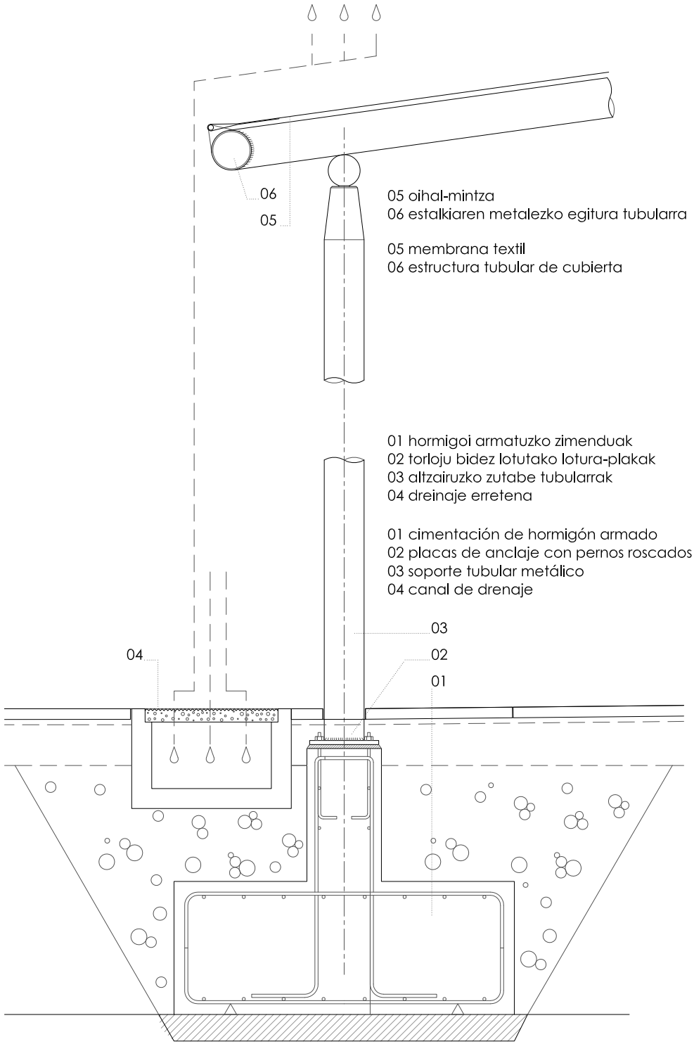
eraikuntza detailea · detalle constructivo
