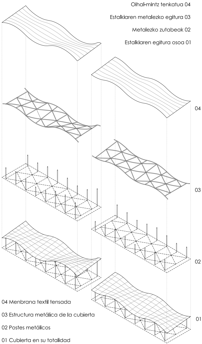
proiektuaren axonometria · axonometría del proyecto
